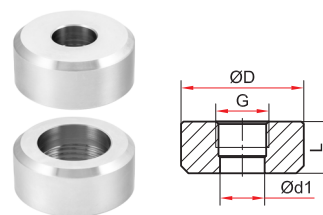
Для датчика давления РПД-И-ФМ с11 №22, №23
