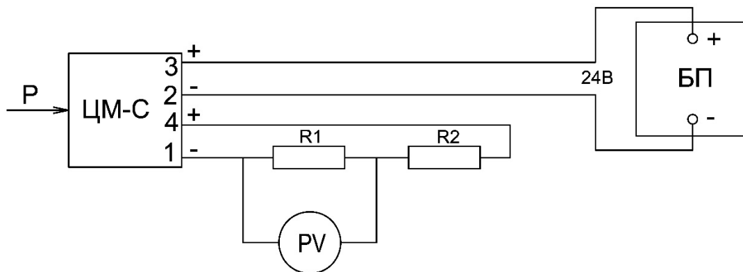
Подключение манометра ЦМ-С
